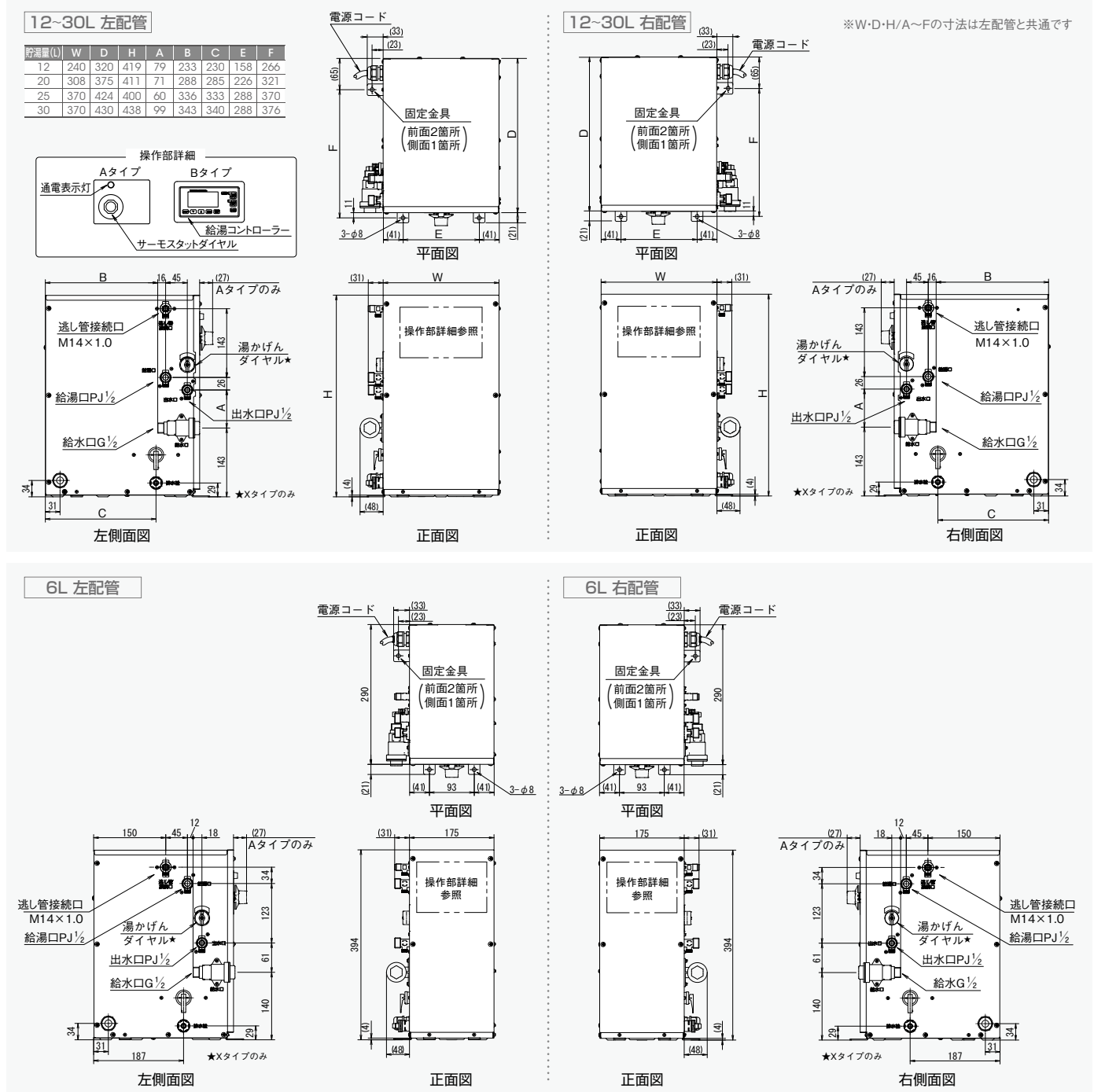
寸法図 ESN
