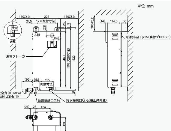
標準配管図
