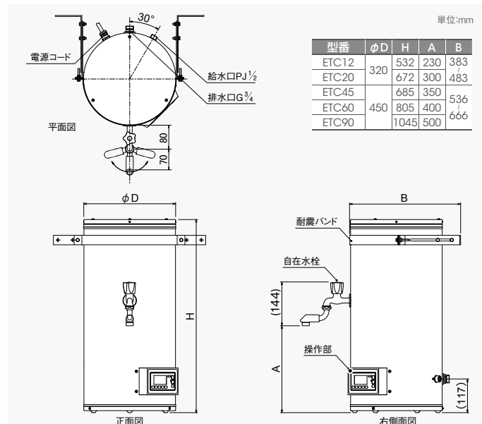
寸法図 ETC
