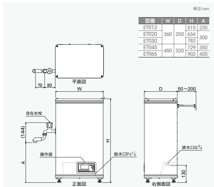
寸法図 ETR
