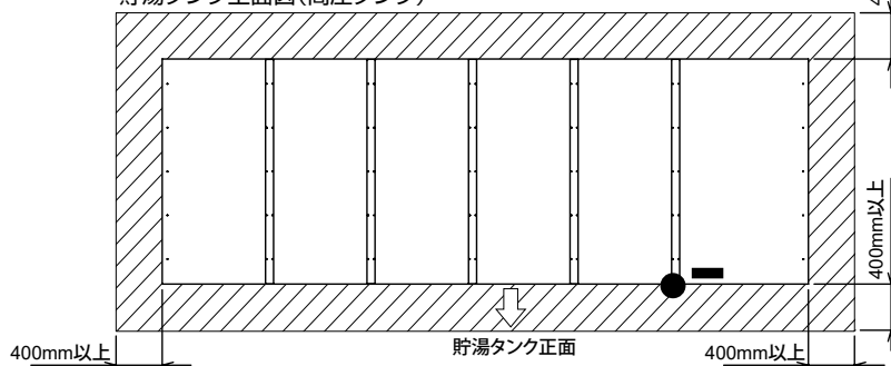
貯湯タンク上面図(高圧タンク)
