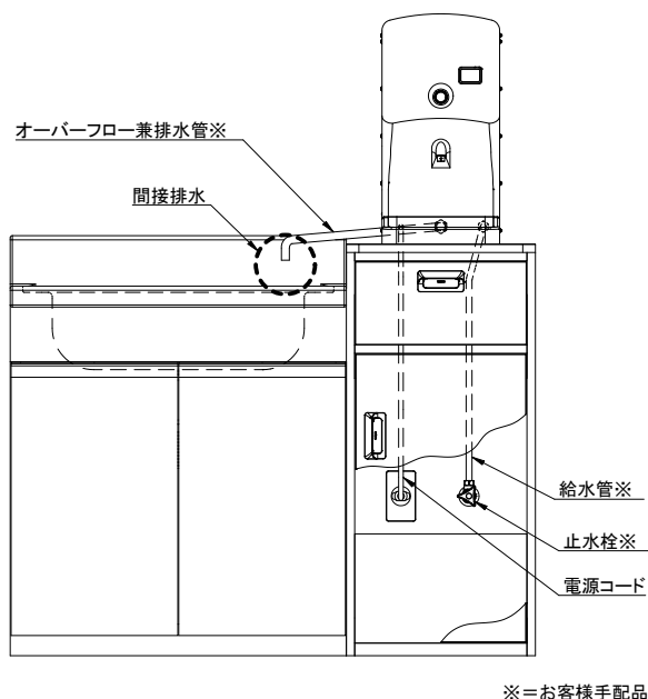
配管施工例
