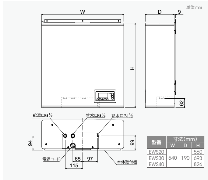
寸法図 EWSシリーズ
