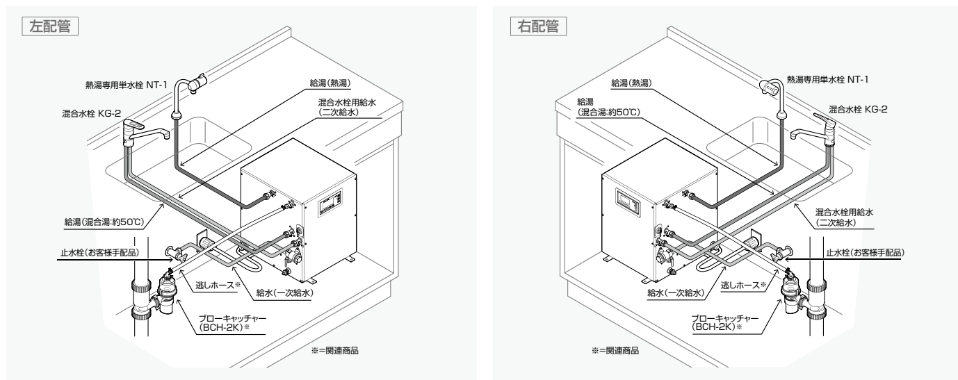
標準配管図
