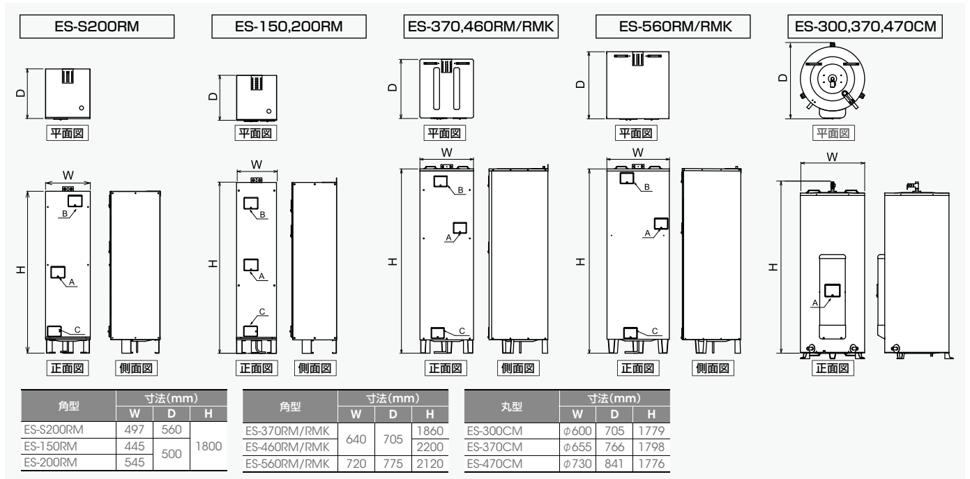
寸法図 A: 漏電ブレーカ点検窓 B: 逃し弁点検窓 C: 排水栓点検窓
