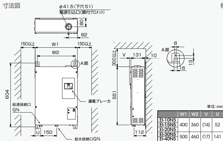
寸法図
