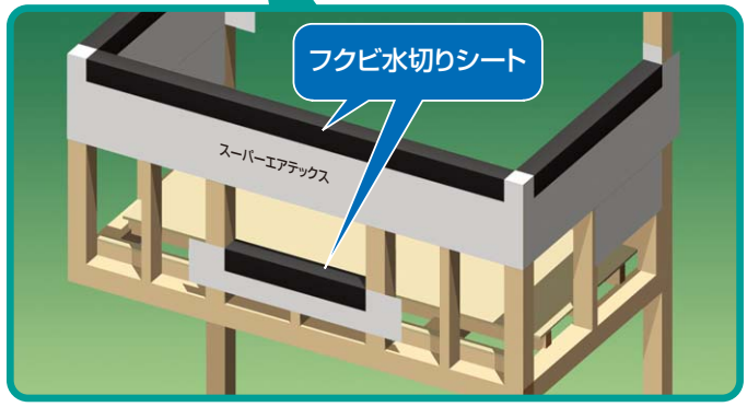
天端全周
