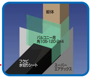
笠木出隅(入隅)部
