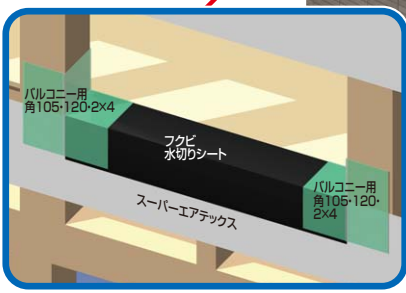
開口下部
