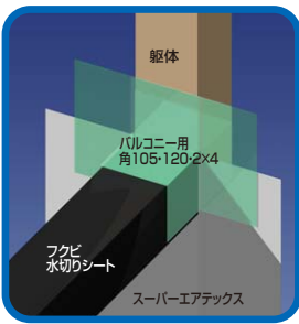
笠木・外壁(直交)
