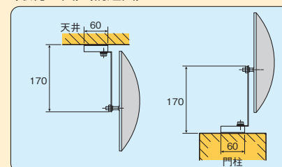
〈取付け図〉〈構造図〉
