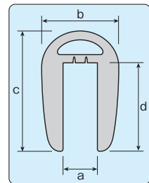
〈構造図〉 H-08~22
