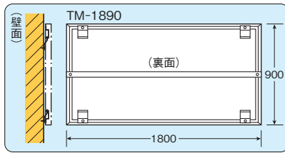
〈取付け図〉〈構造図〉
