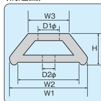
〈構造図〉
