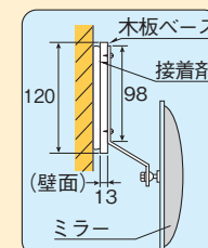
〈取付け図〉〈構造図〉
