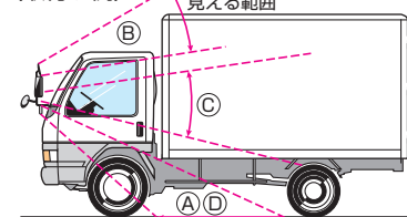
〈取付け例〉
