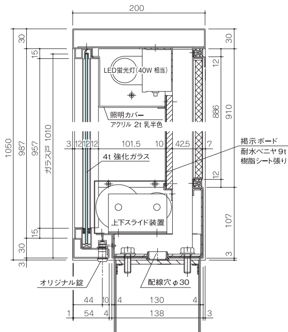
立断面
