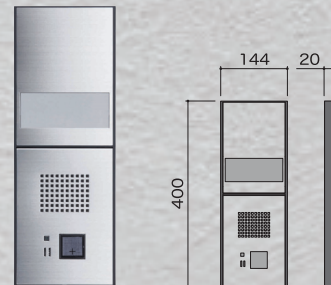
●スリムポートS (室名札・インターホンパネル) ¥7,500
