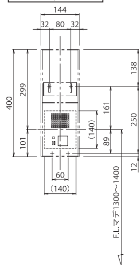
スリムポーチ S
