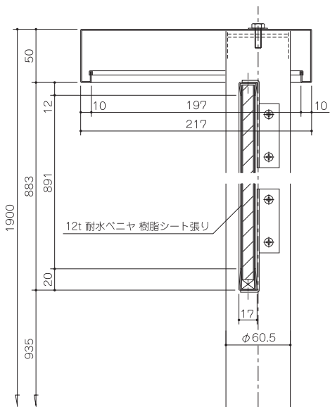
立断面
