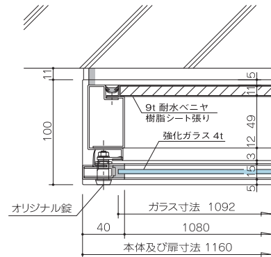
平断面
