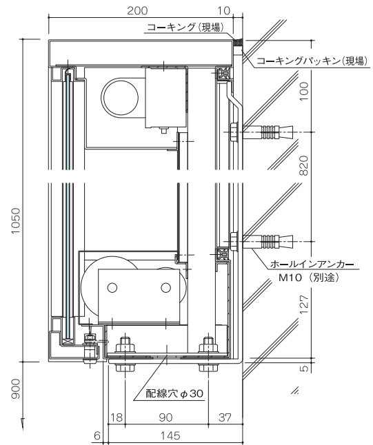
立断面
