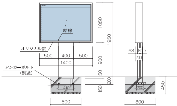
立断面
