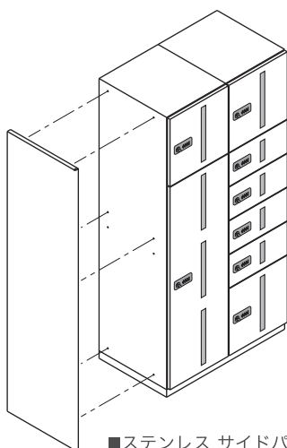
■ステンレス サイドパネル ステンレス (SUS304) 0.8t ヘアライン仕上 クリアー焼付塗装
