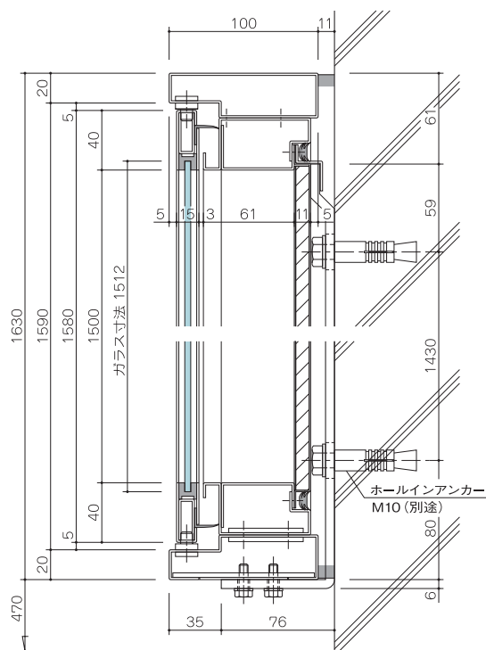
立断面
