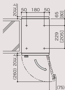
●FX-CB・[49]-HL ※[]はFX-CB49-HL
