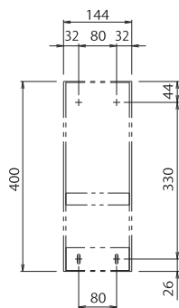
スリムポーチ N
