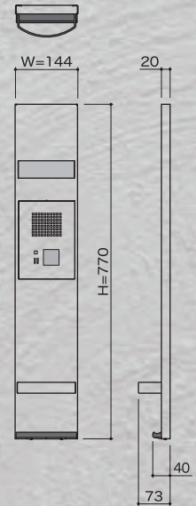
●ドアフレンド3S (ハイブレーション仕上) ¥19,000
