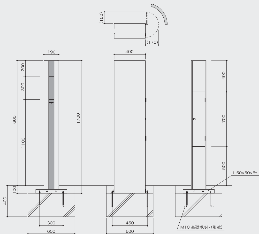
■ 詳細図
