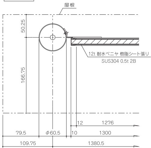
平断面
