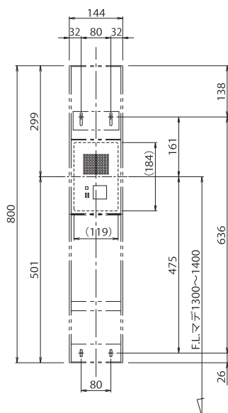
スリムポーチ T
