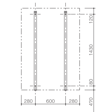
アンカーピッチ図
