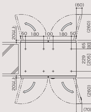
●FX-RB・[49]-HL ※[]はFX-RB49-HL
