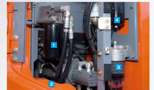
1 エンジンオイルフィルタ 2 パイロットフィルタ 3 燃料プレフィルタ 4 燃料メインフィルタ
