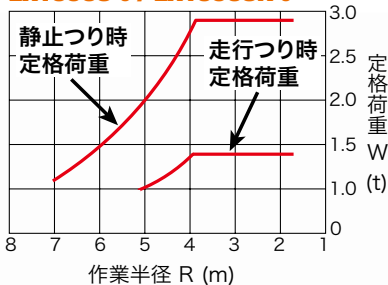
ZX135US-6 / ZX135USK-6
