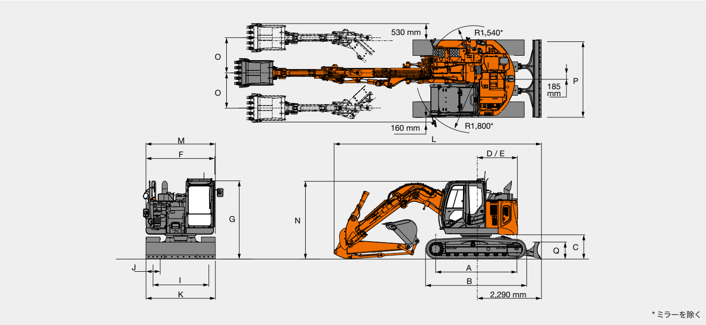
寸法図
