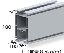
L (質量 8.5kg/m)
