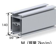
M (質量 7kg/m)
