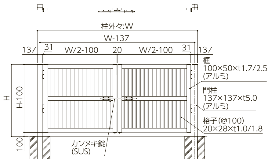
■大型門扉A型〈両開き〉サイズ表
