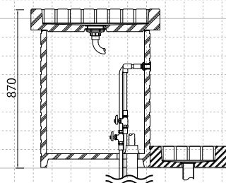
シャワープレイス ショートタイプ レトロブリック
