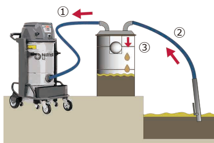
図 1 汚水回収の流れ
