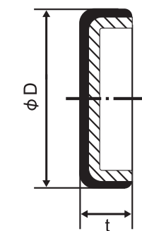
SC-N型 (外周ツバ無し)
