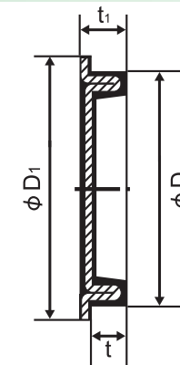
SC-A型 (外周ツバ付)
