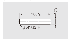
【取付穴加工図】
